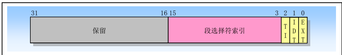
图 4-31 错误码格式
