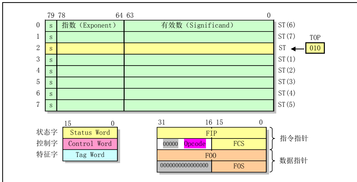
图 11-5 80387 的寄存器
