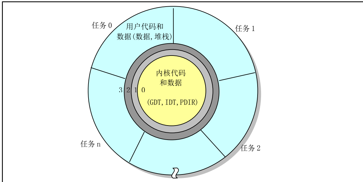
图 5-13 多任务系统
